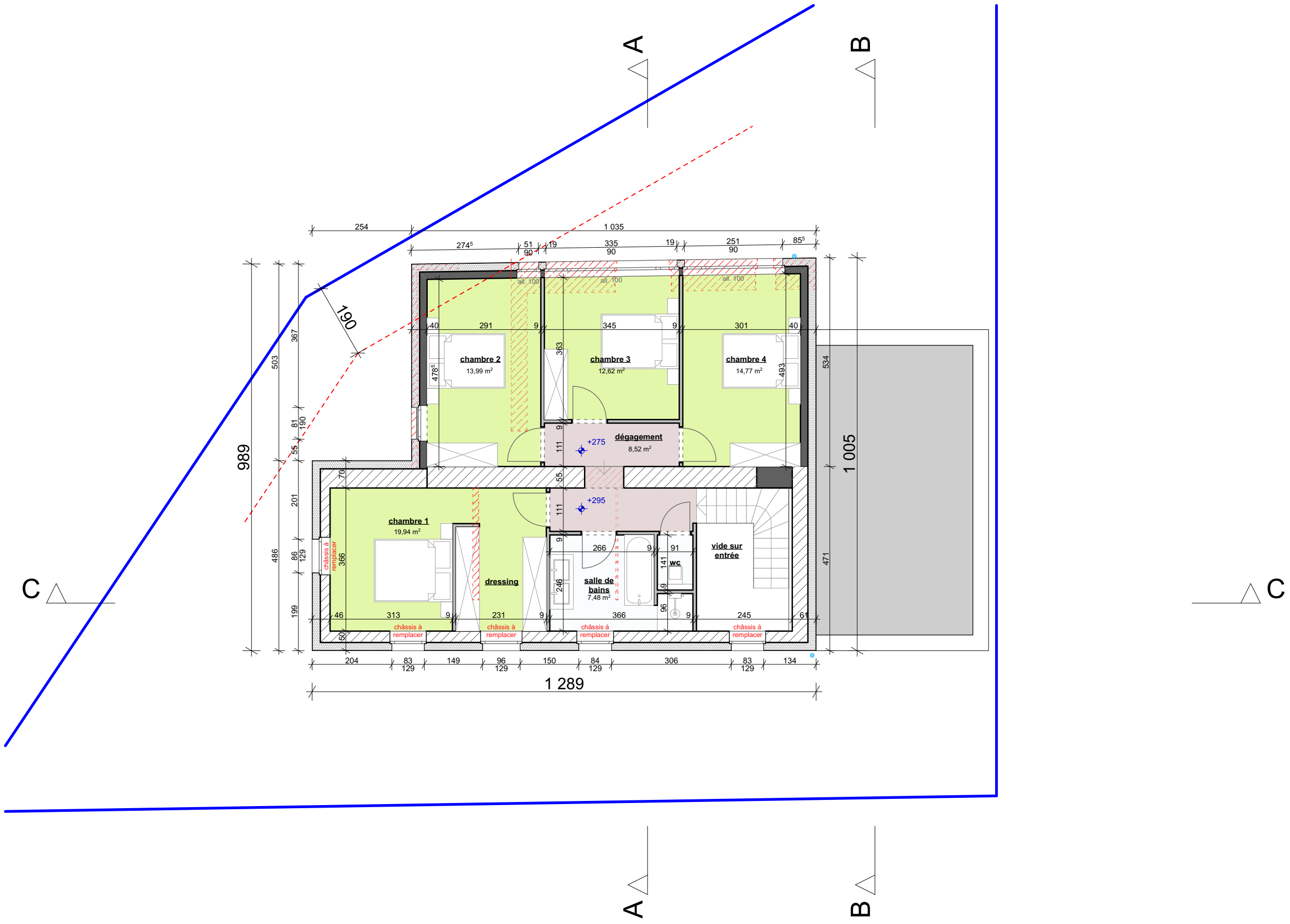
PLAN 1° ETAGE - NIVEAU +295
